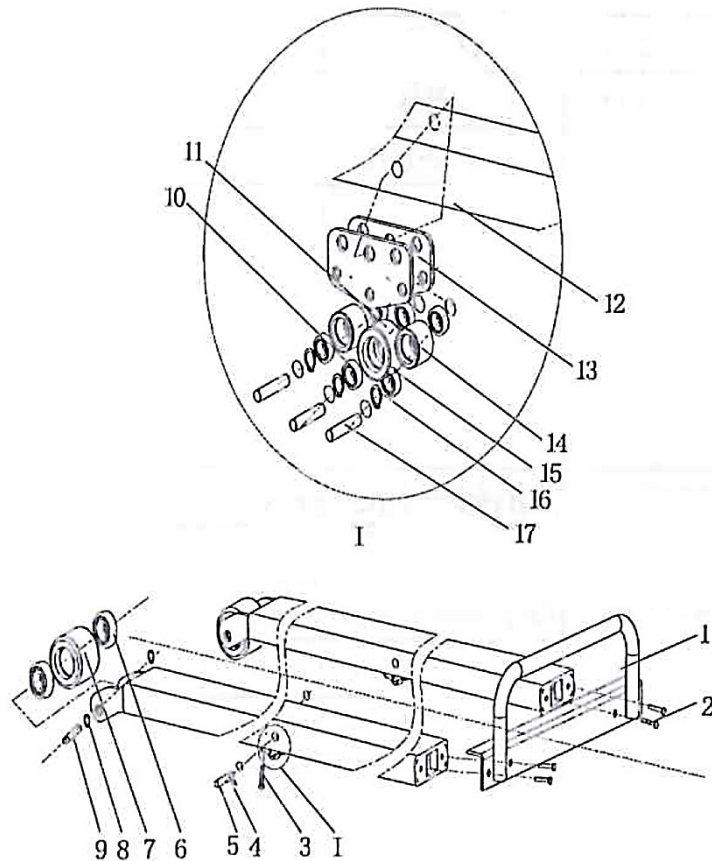
Взрыв схема 4
