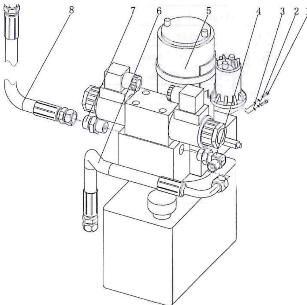
Взрыв схема 1.
