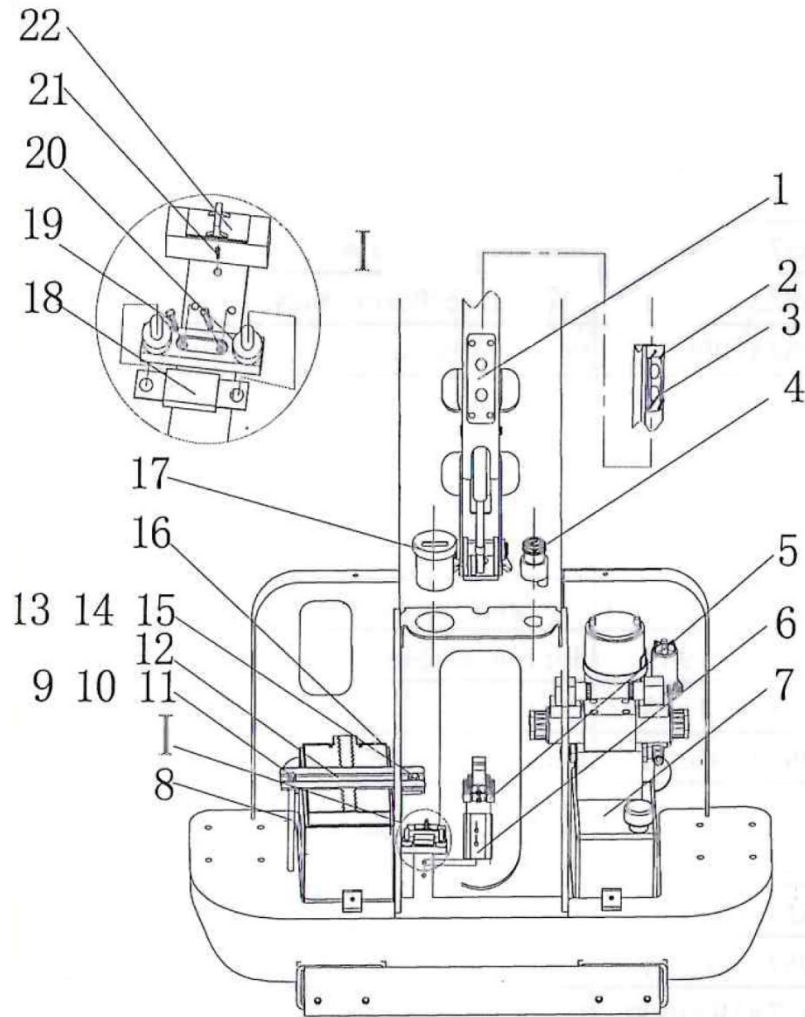
Взрыв схема 2
